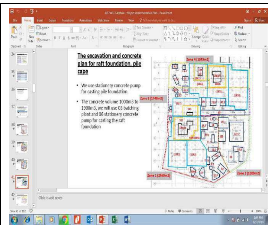
Plan to pour concrete for Big foundation
